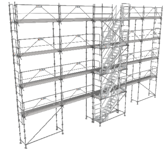
ÉCHAFAUDAGES FIXES
